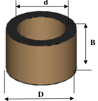
Cartouche (Élément de rechange)
